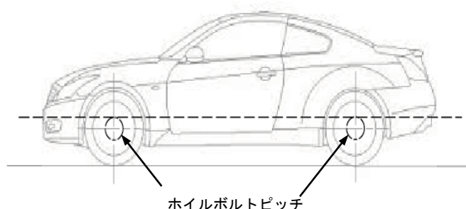
破線面より下の前後オーバーハング部は形状変更可 (図 11-1)
